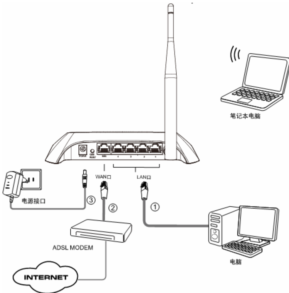
图 4-1 TL-WR742N 硬件安装示意图
