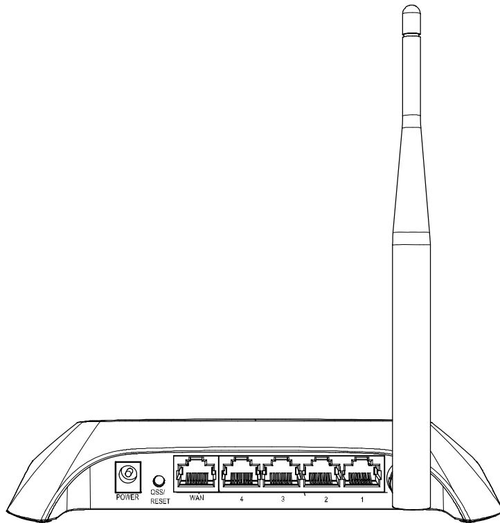
图 3-2 TL-WR742N 后面板示意图
