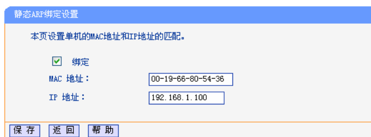
图 5-50 添加静态 ARP 绑定条目
